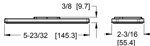
Optional Deckplate
