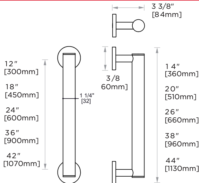
Grab Bar 12"/18"/24"/36"/42" SYD-GB3-12/18/24/36/42
