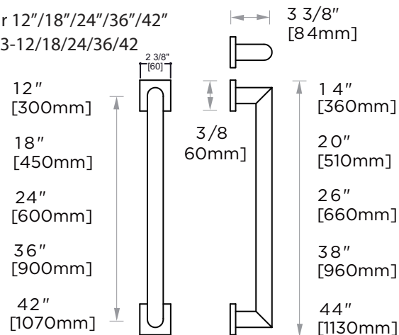
Grab Bar 12"/18"/24"/36"/42" SYD-GB5-12/18/24/36/42
