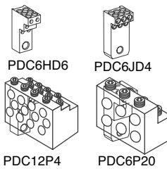
R-Frame Compression Lug Kit
