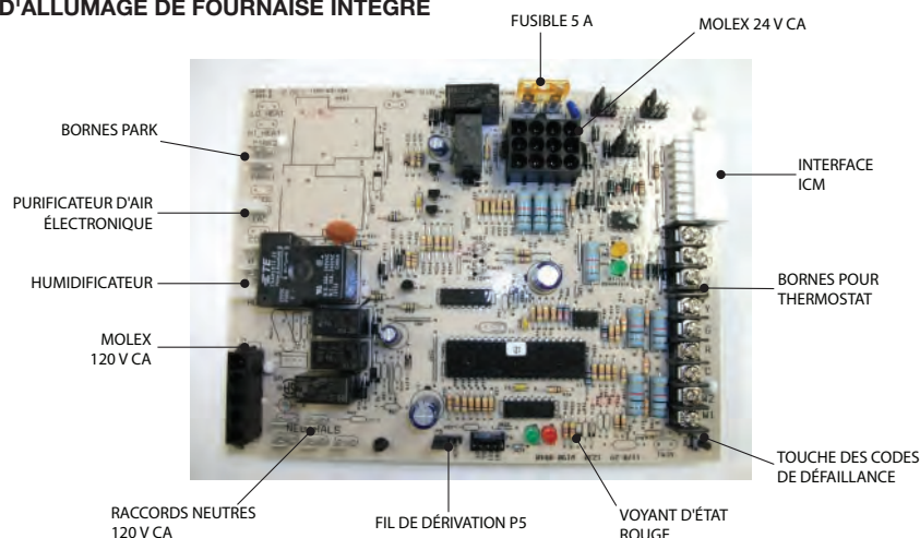
FIGURE 36 - CONTRÔLE D'ALLUMAGE DE FOURNAIE INTÉGRÉ
