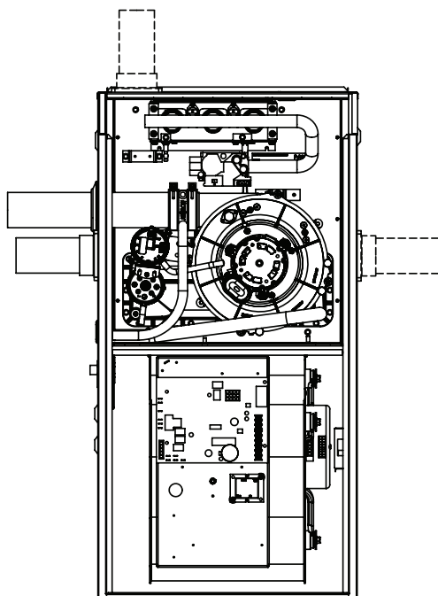
FIGURE 16 - OPTION D'ÉVACUATION ET DE VIDANGE ASCENDANTE
