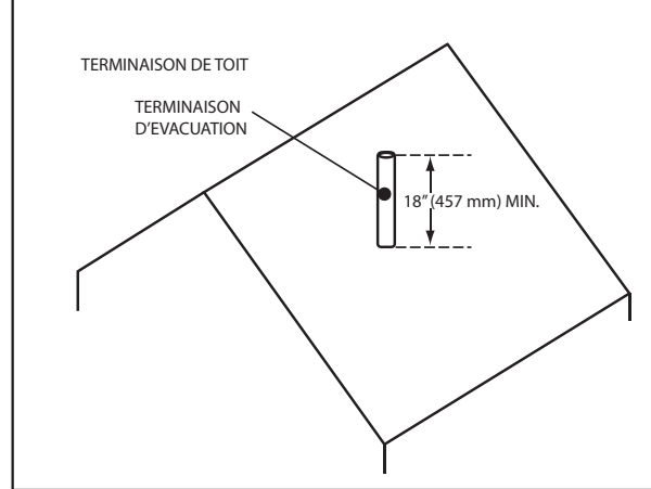
FIGURE 10 - ÉVACUATION VERTICALE
