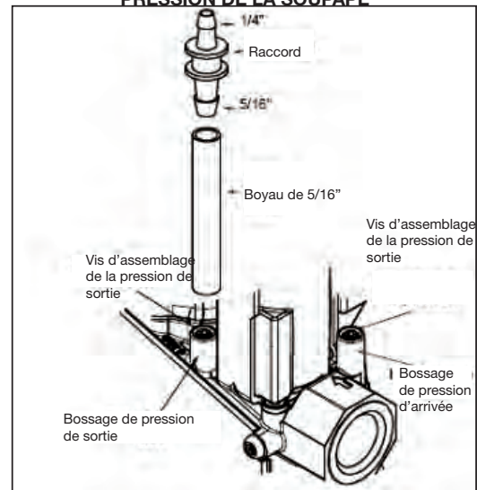
FIGURE 32 - ENSEMBLE DE VÉRIFICATION DE LA PRESSION DE LA SOUPAPE
