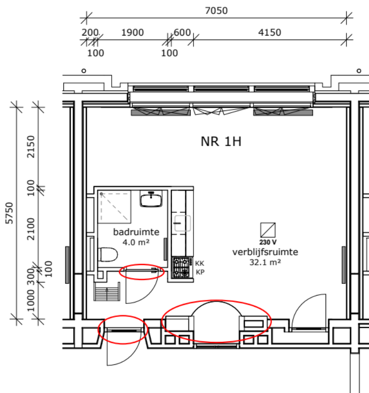
1e verdieping 1 : 100
