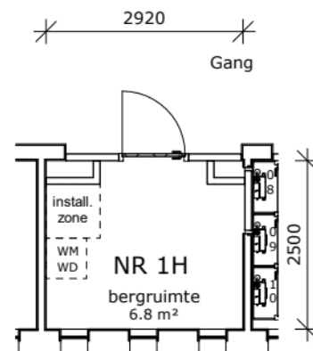
1e verdieping 1 : 100
