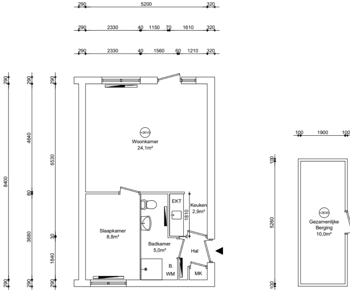
Appartement GO wonen 43,68m 2
