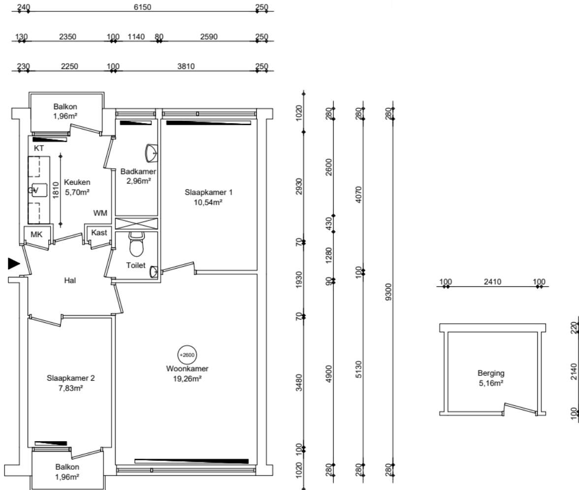
Appartement GO wonen 54,67m 2
