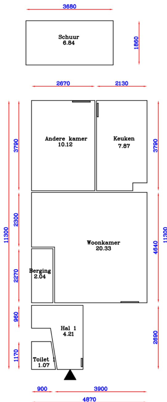
Begane grond
