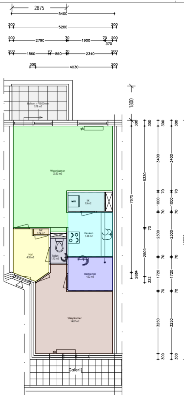
Verdieping_4e
