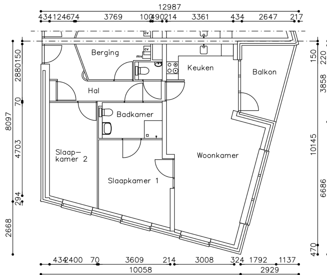
3e verdieping
