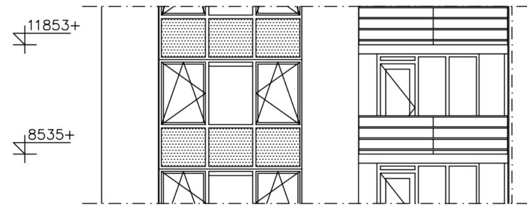
Zijgevel
