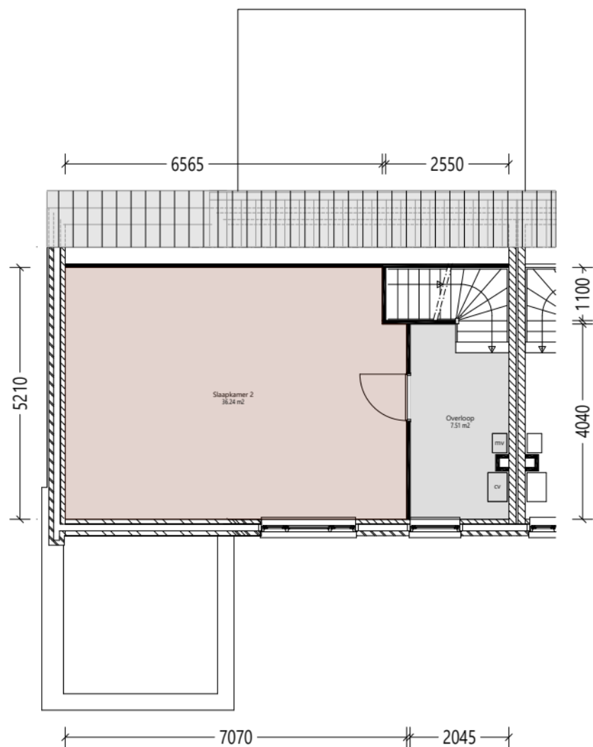
Verdieping_1e
