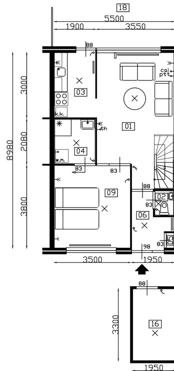
BEGANE GROND
