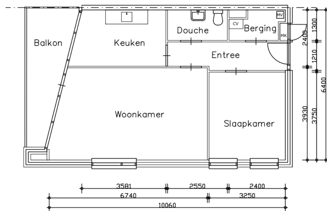
Plattegrond
