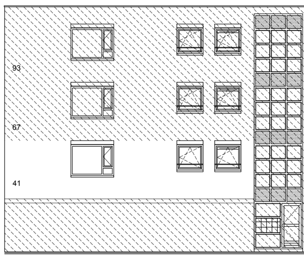
Zijgevel
