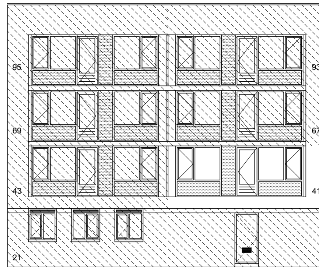
Kopgevel
