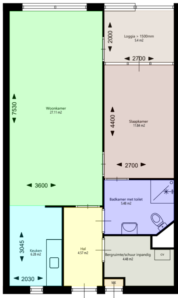
Verdieping_3e
