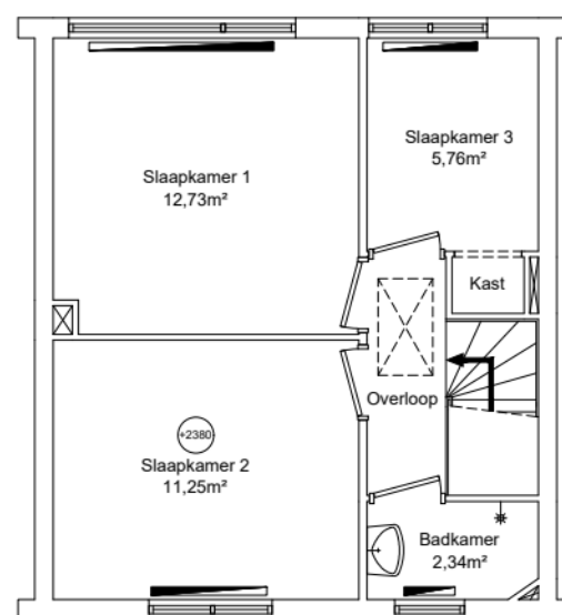
1e verdieping GO wonen 38,67m²
