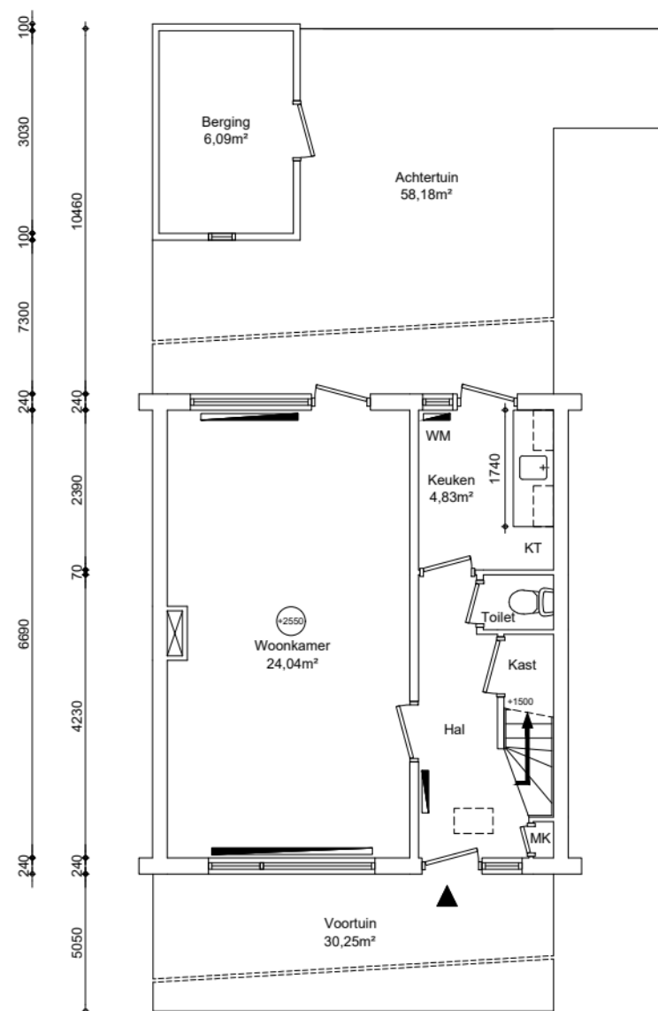
Begane grond GO wonen 38,67m²
