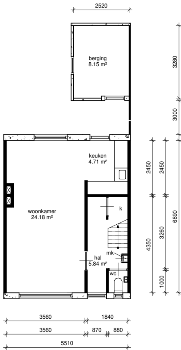
begane grond
