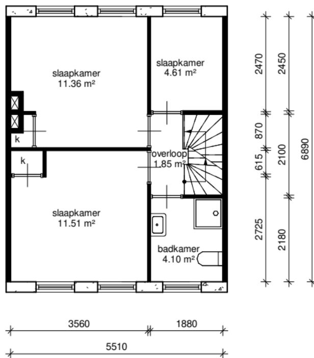
eerste verdieping
