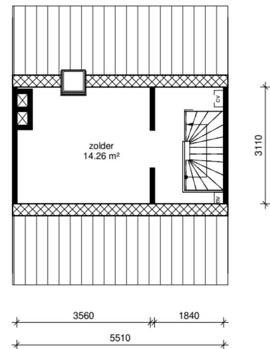
tweede verdieping
