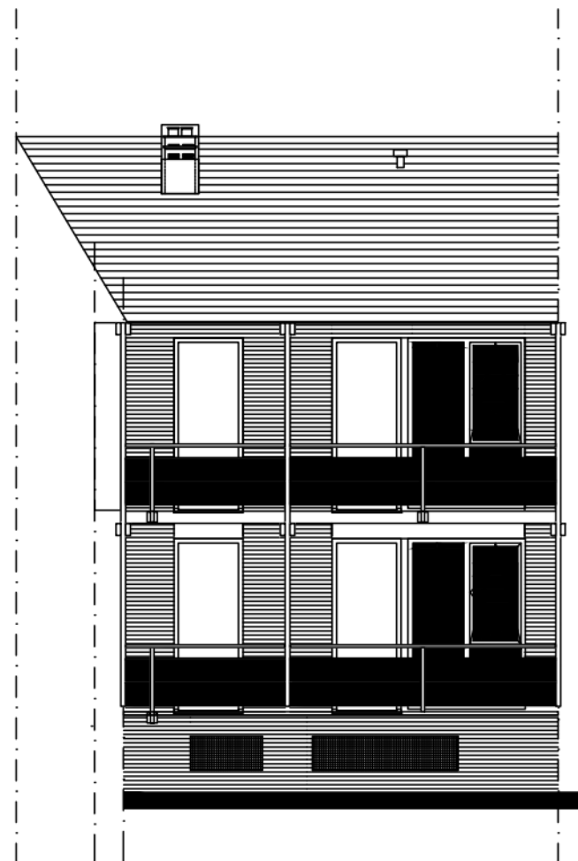
Voorgevel
