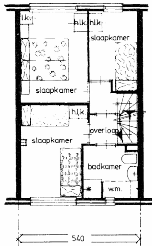
1 e VERDIEPING
