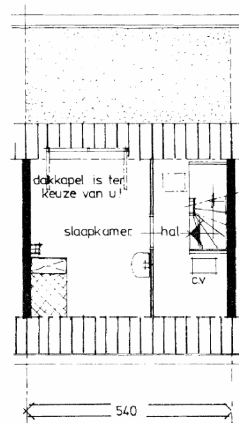
AFGEBOUWDE ZOLDER
