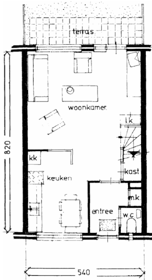
BEGANE GROND
