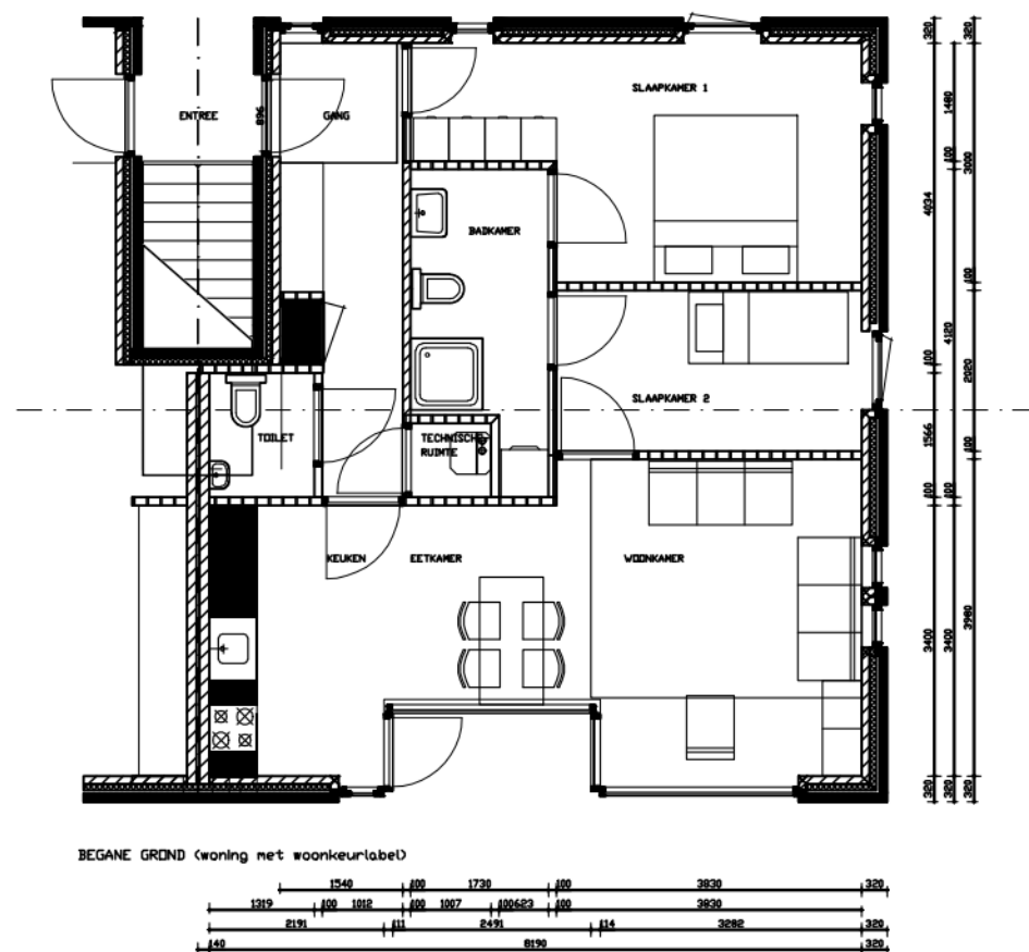
Beganegrond
