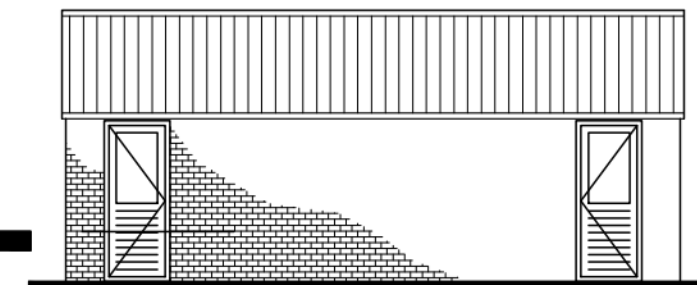
Achtergevel
