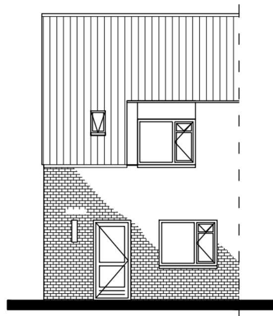
Voorgevel
