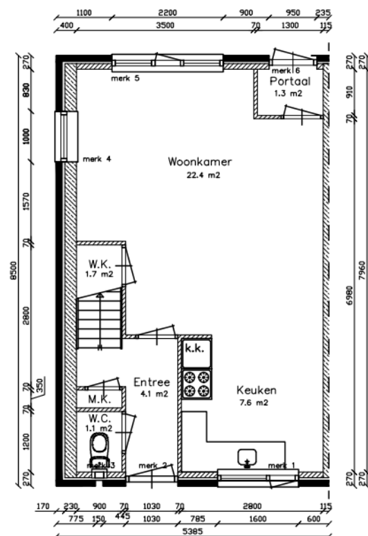
Beganegrond
