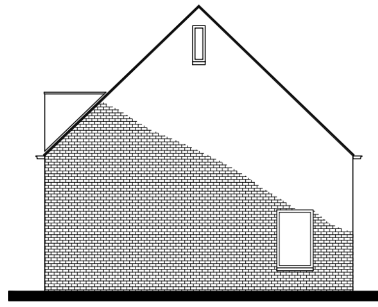
Zijgevel
