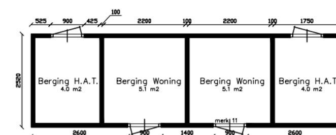
Platte-grond
