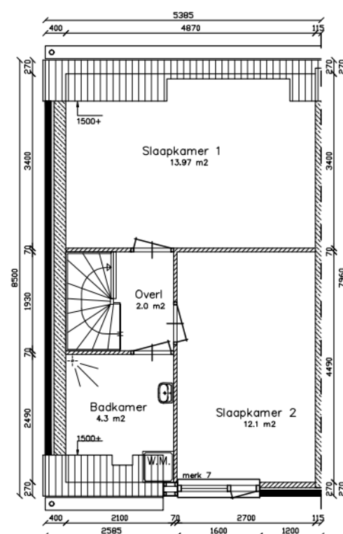
Verdieping
