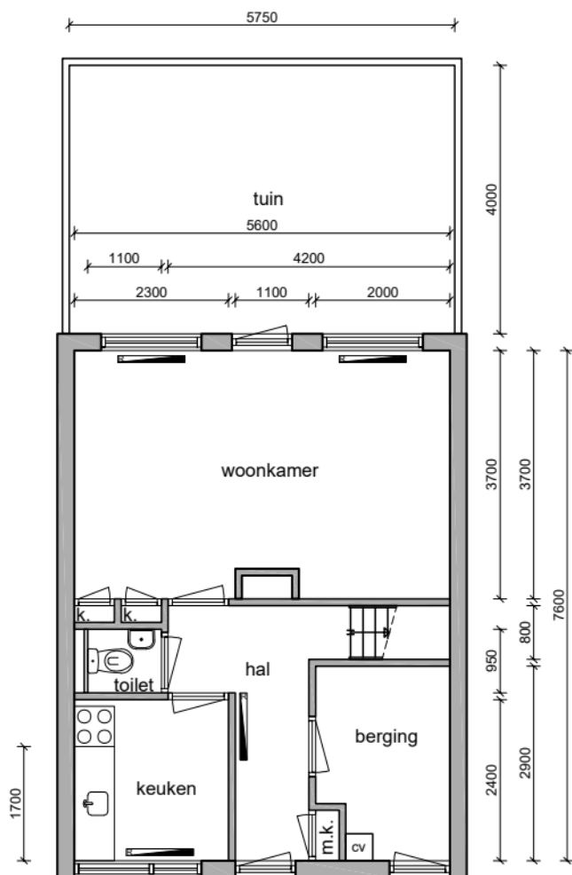
Begane grond
