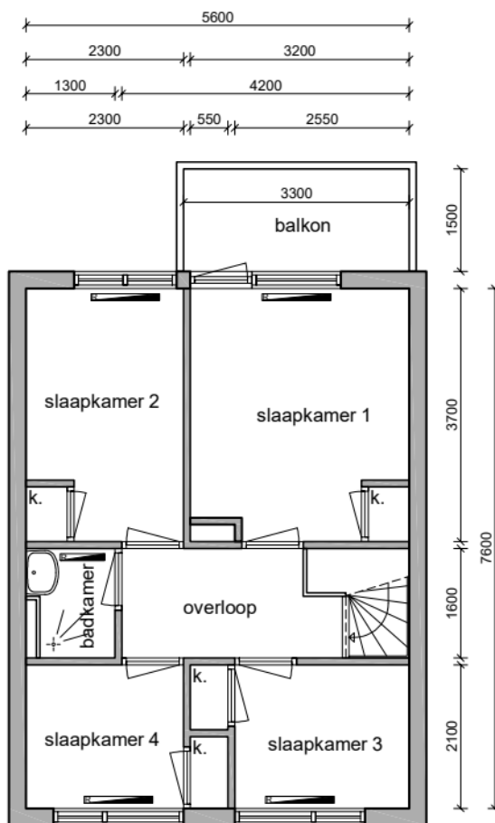
1e verdieping
