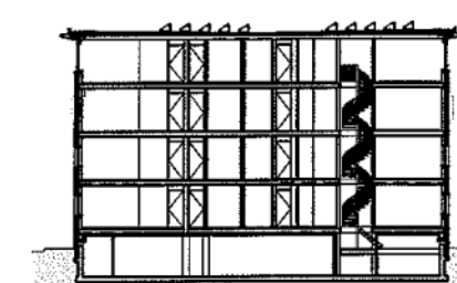
DOORSNEDE
