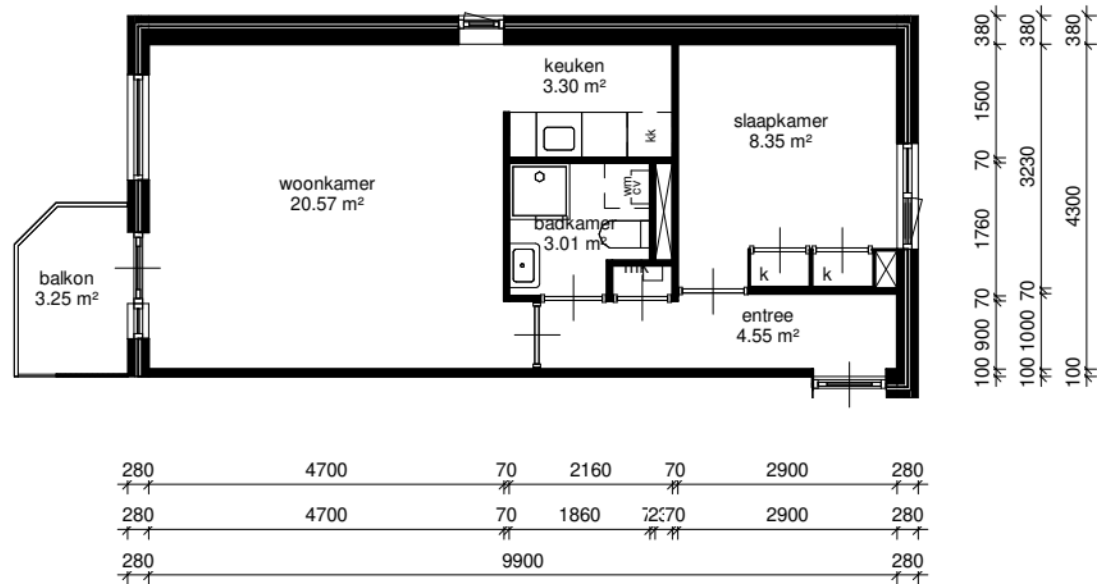
eerste verdieping
