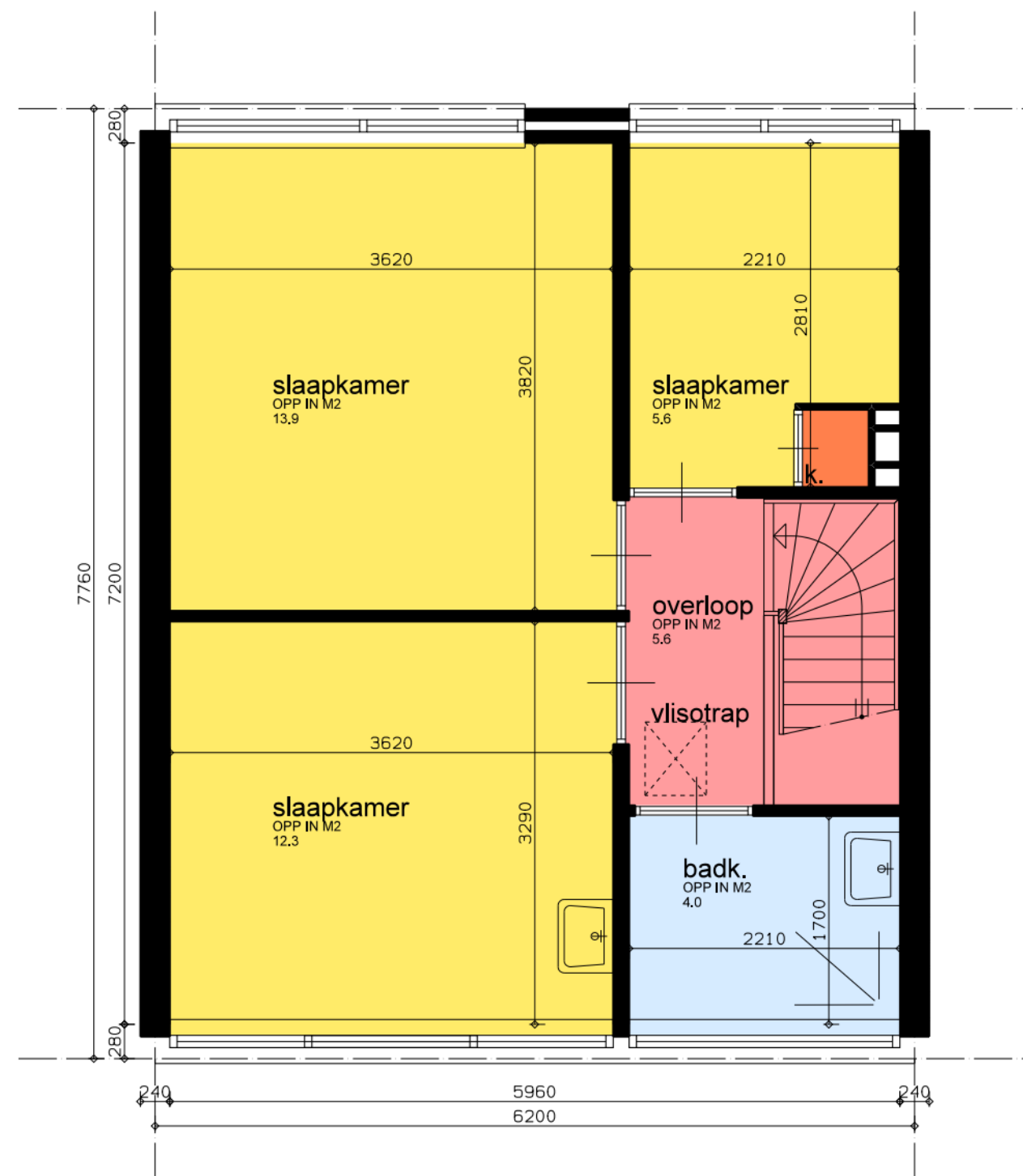
eerste verdieping
