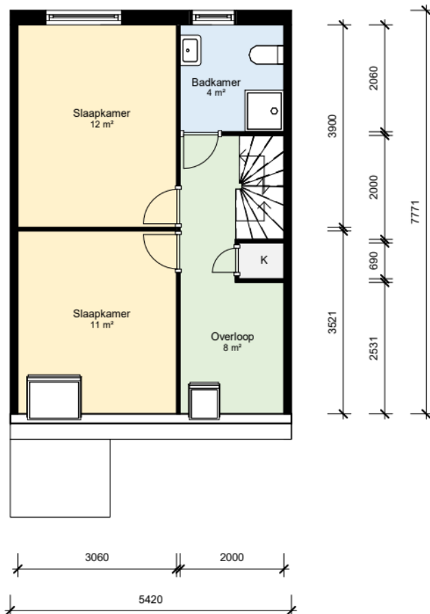
01 Eerste verdieping
