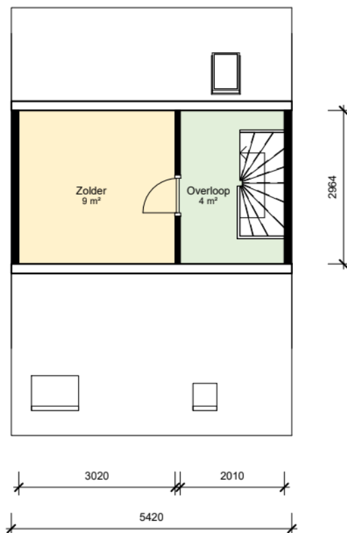
02 Tweede verdieping
