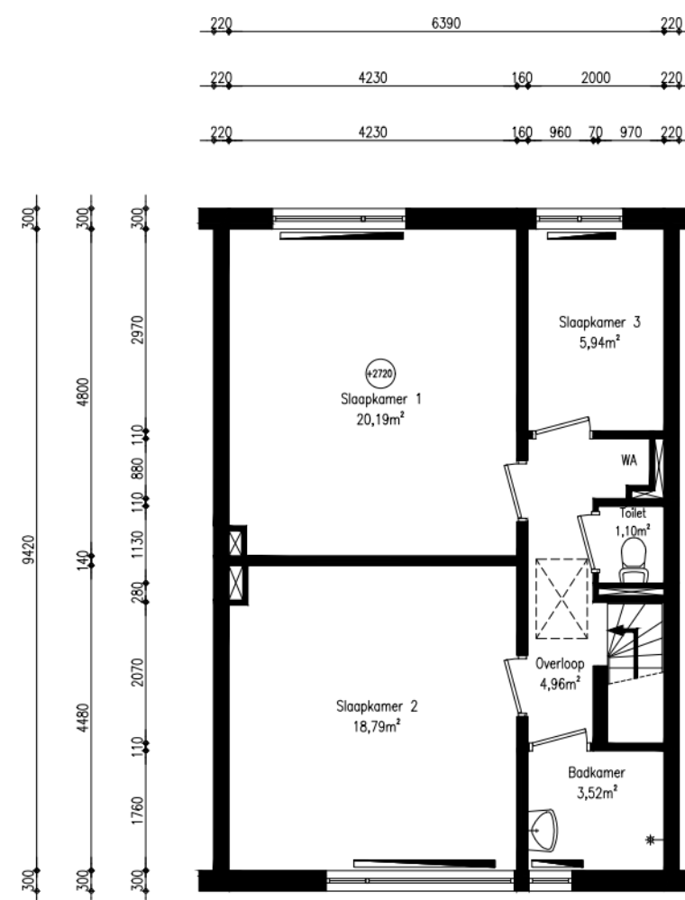
1e verdieping
