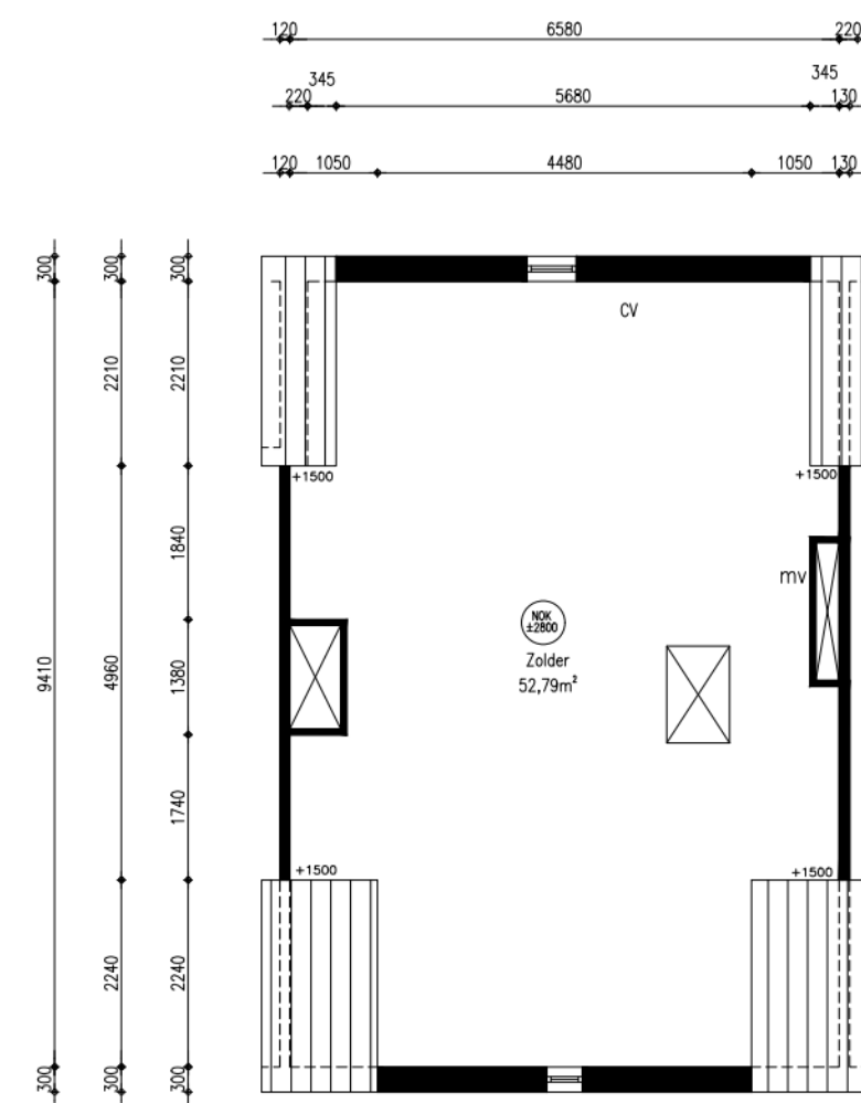
2e verdieping
