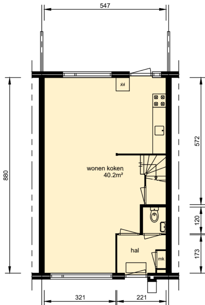
begane grond
