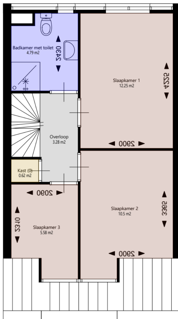
Verdieping_1e
