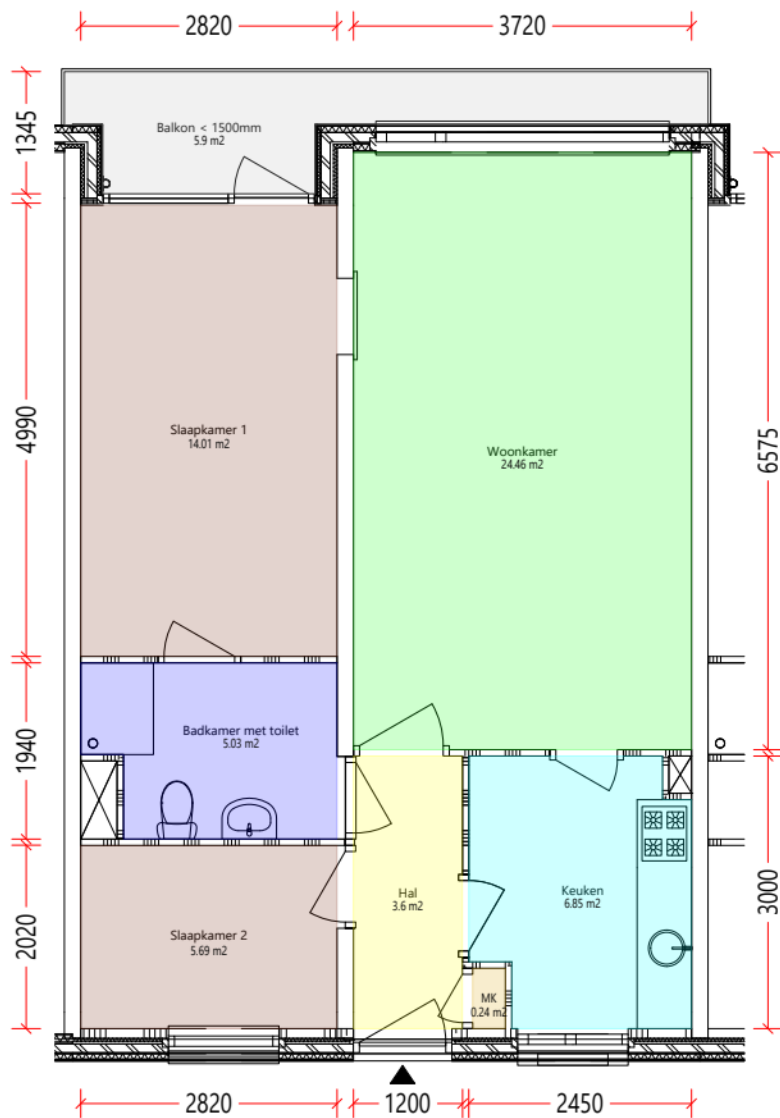
Verdieping_1e
