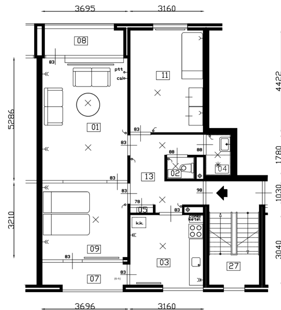
PLATTEGROND
