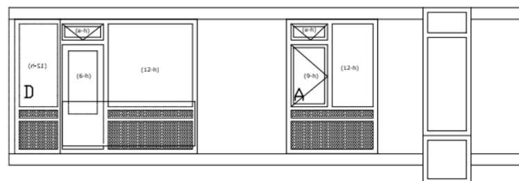
LINKERZIJGEVEL
