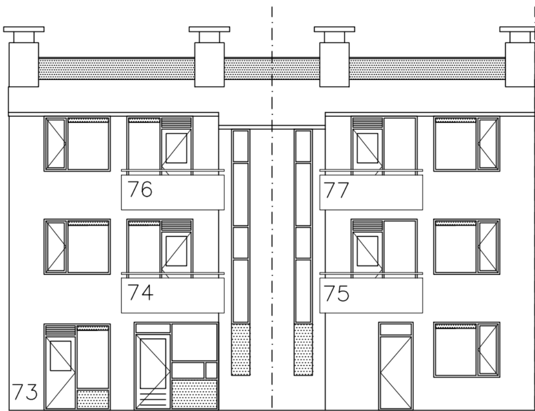
Vooraanzicht
