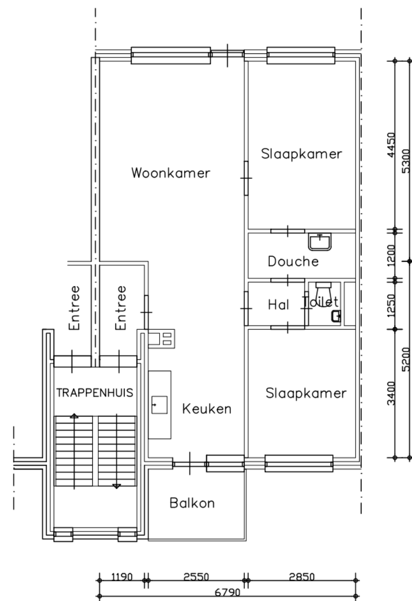
Plattegrond
