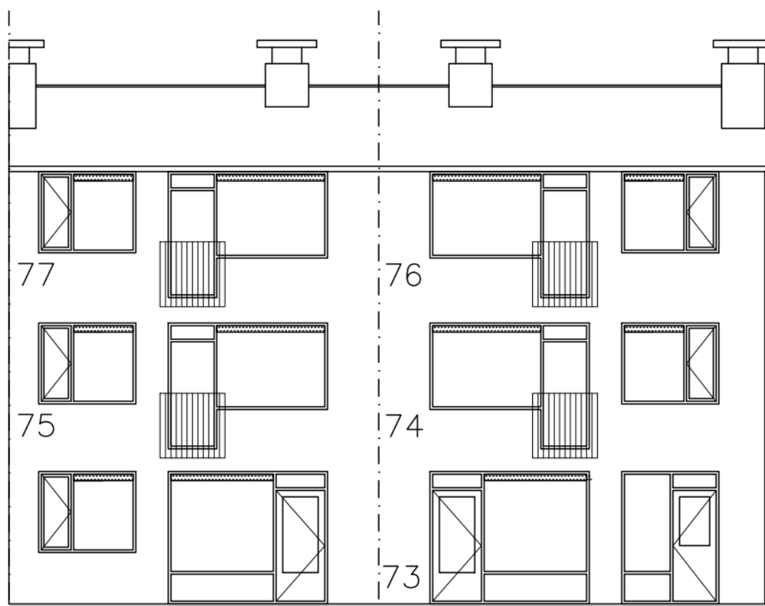
Achteraanzicht
