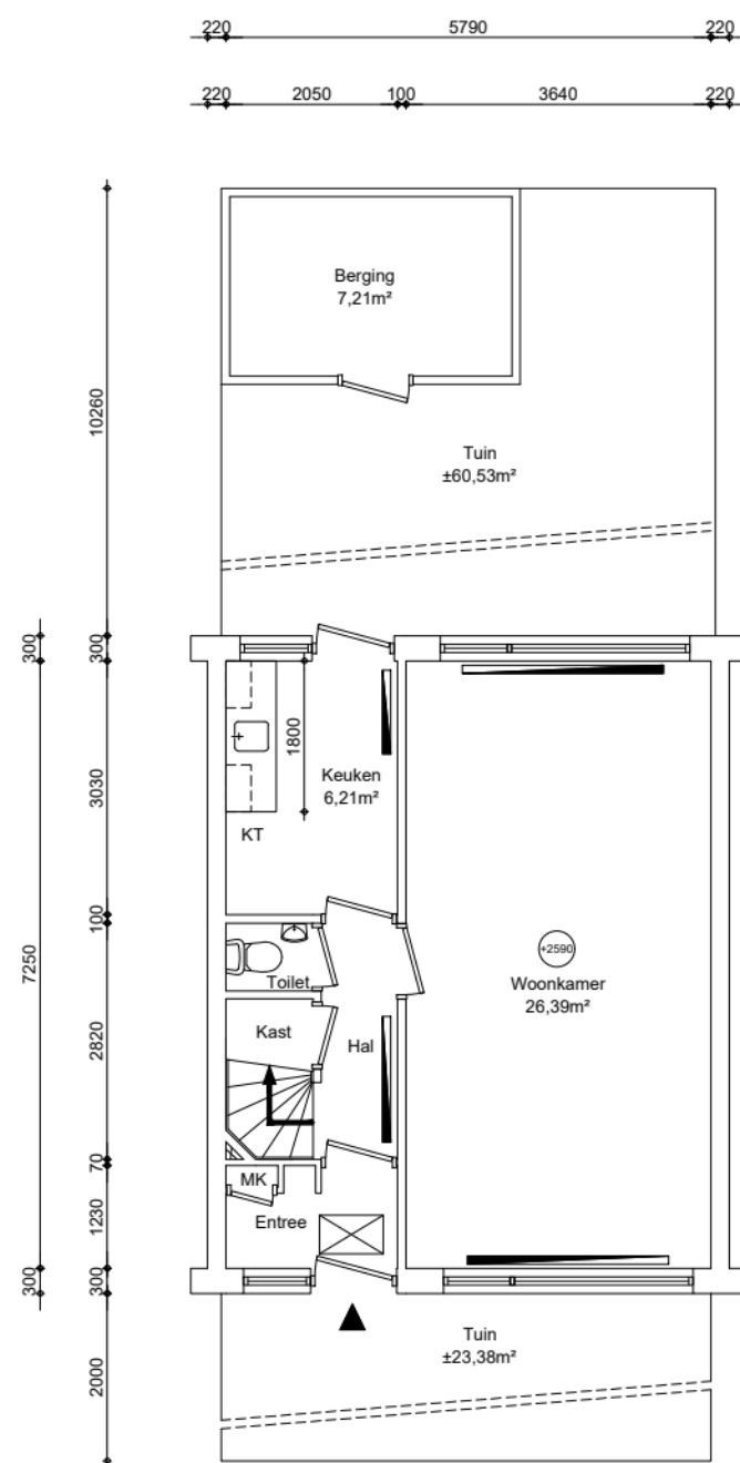
Begane grond GO wonen 41,98m²
