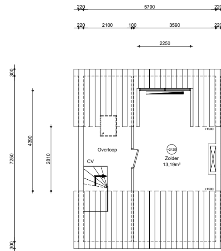
2e verdieping GO wonen 19,82m²
