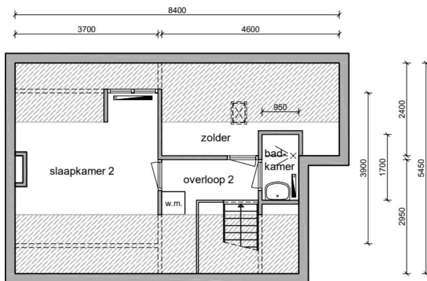
2e verdieping
