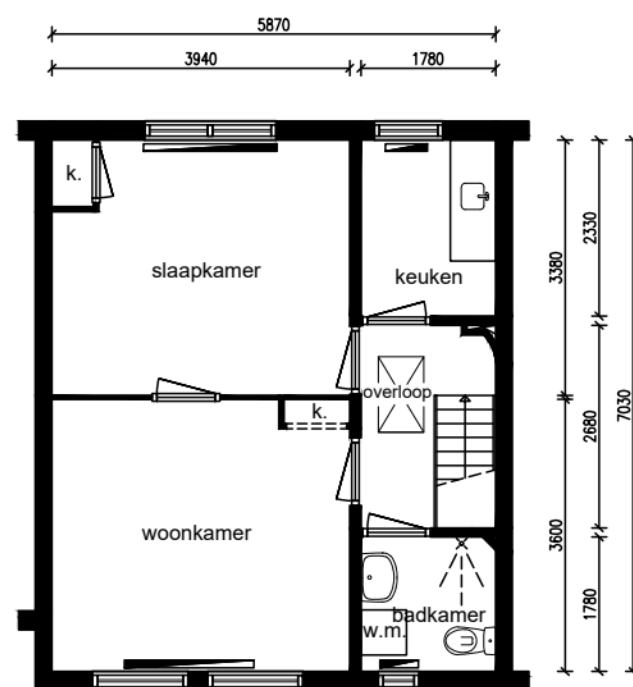
1e verdieping
