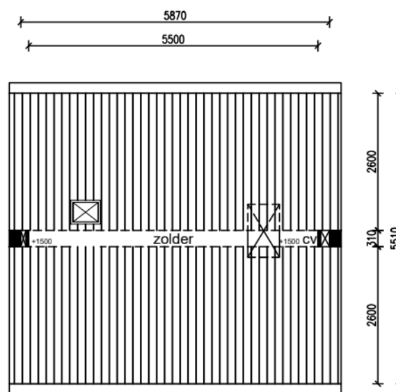
2e verdieping
