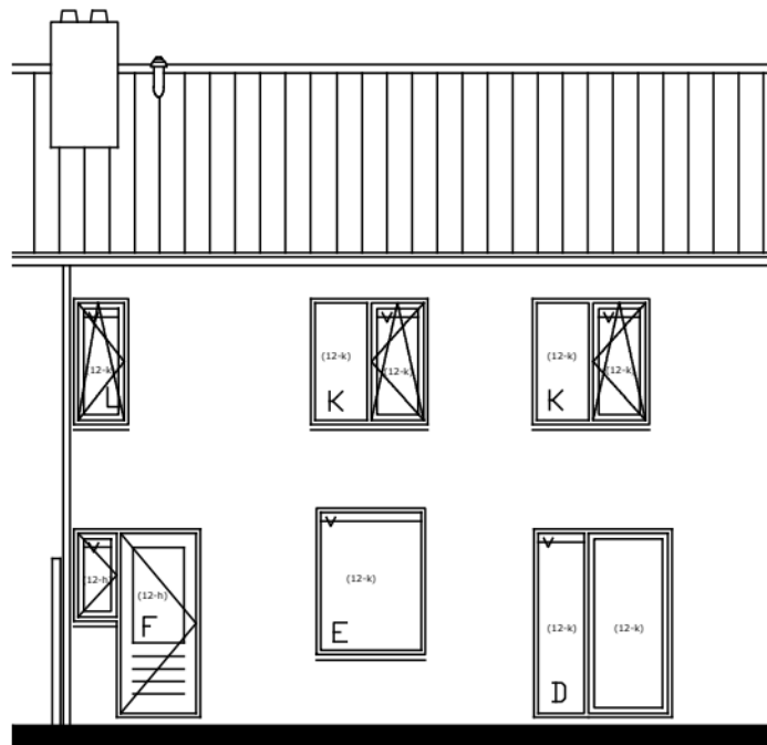
ACHTERGEVEL
