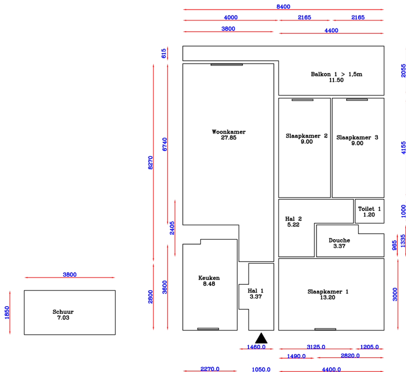
Begane grond
