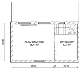
4e Verdieping
