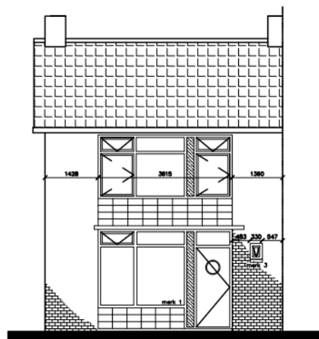
Voorgevels
