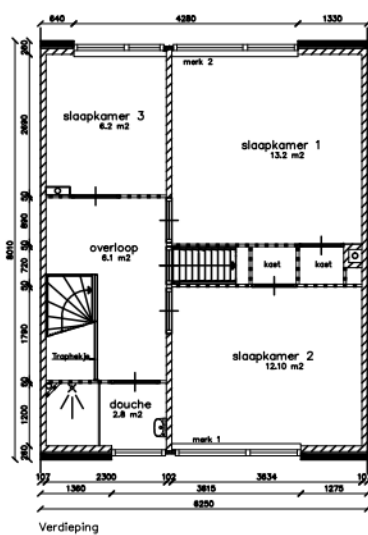
Verdieping
