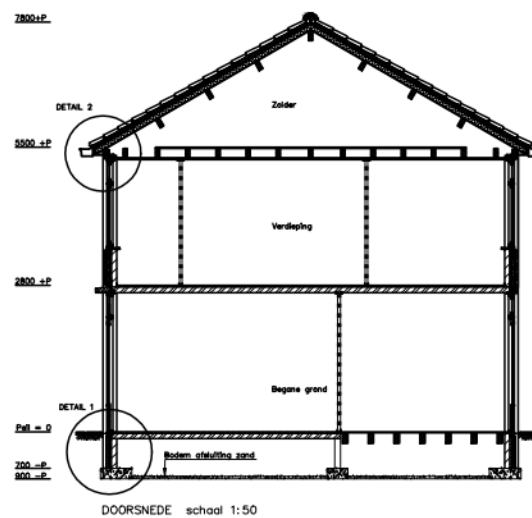
DOORSNEDE schaal 1:50
