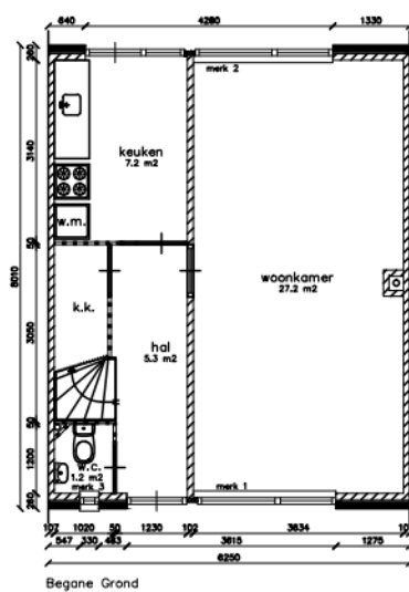
Begane Grond
