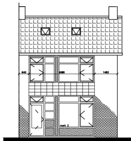
Achtergevels
