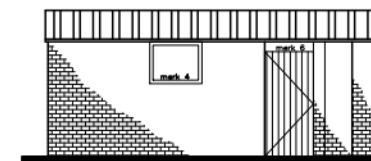
Voorgevel Schuur
