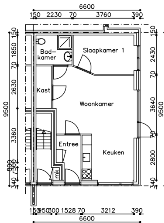
Begane grond
