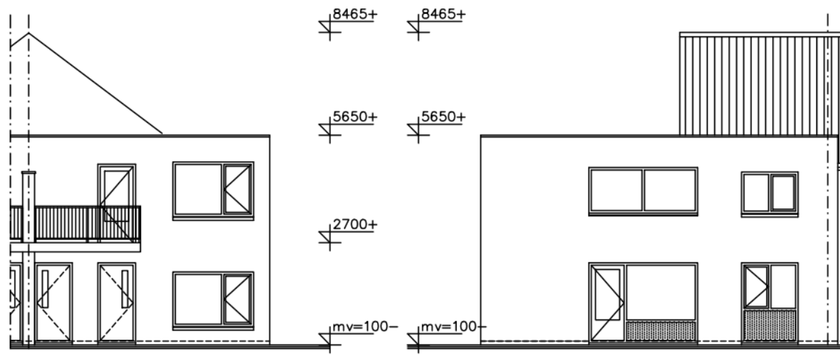
Voorgevel
