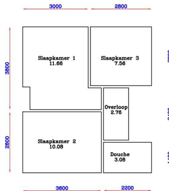
1e Verdieping
