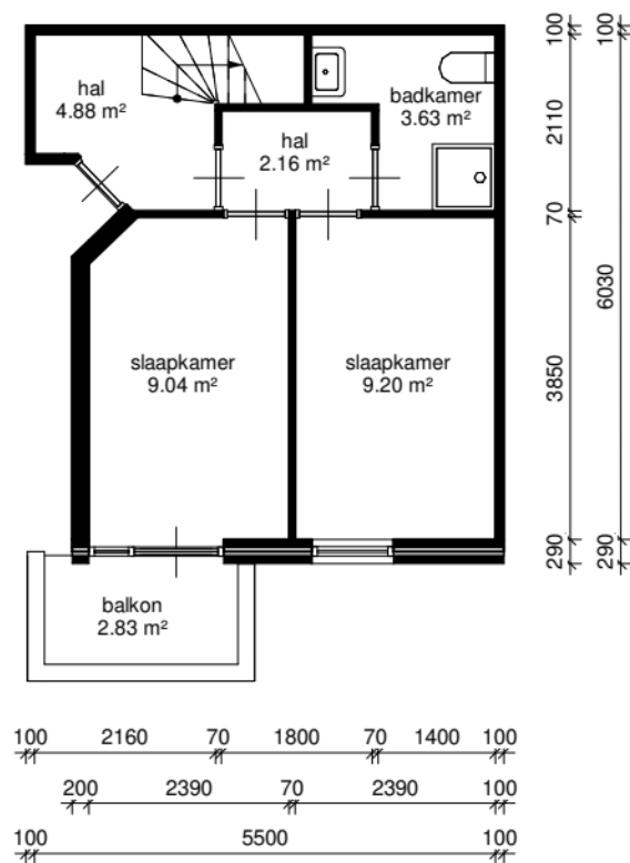
eerste verdieping
