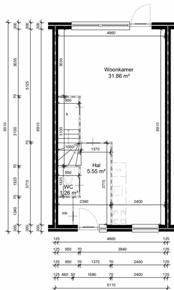
Begane grond
