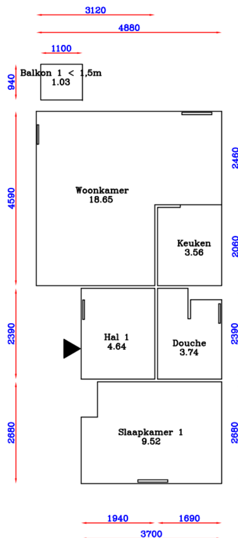
2e Verdieping
