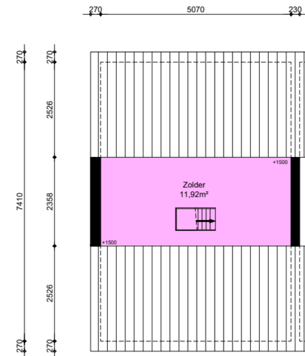
2e verdieping
