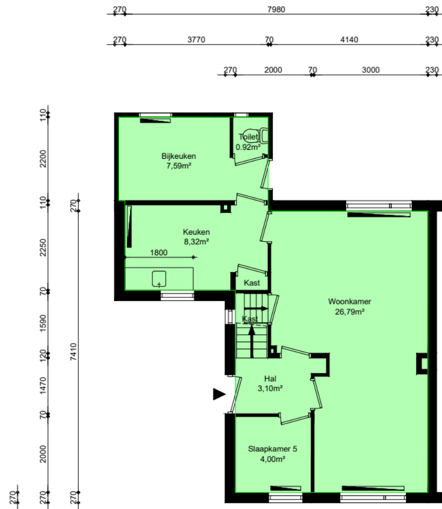
Begane grond
