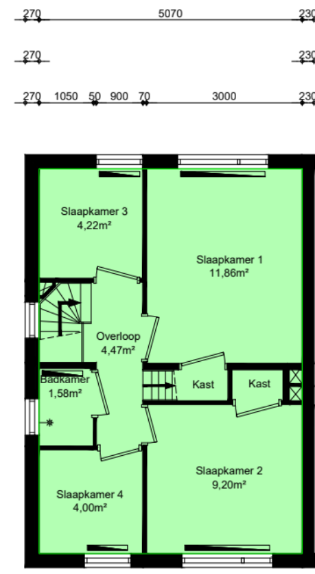
1e verdieping
