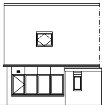
Voorgevel
