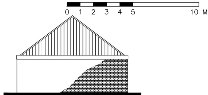
Rechter kopgevel
