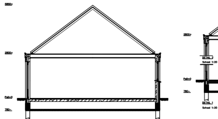
Doorsnede
