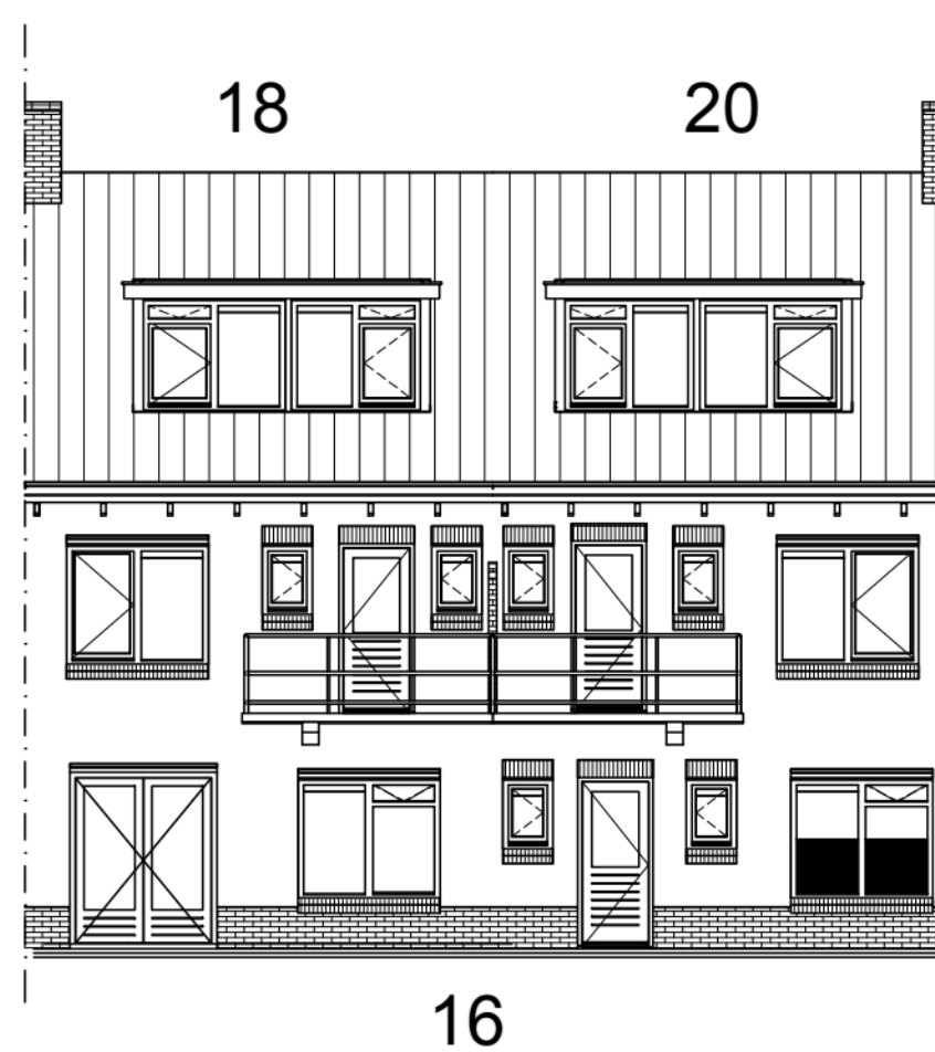
Achteraanzicht
