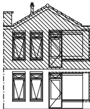
Achtergevel
