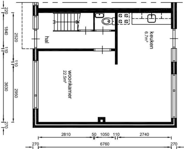
begane grond
