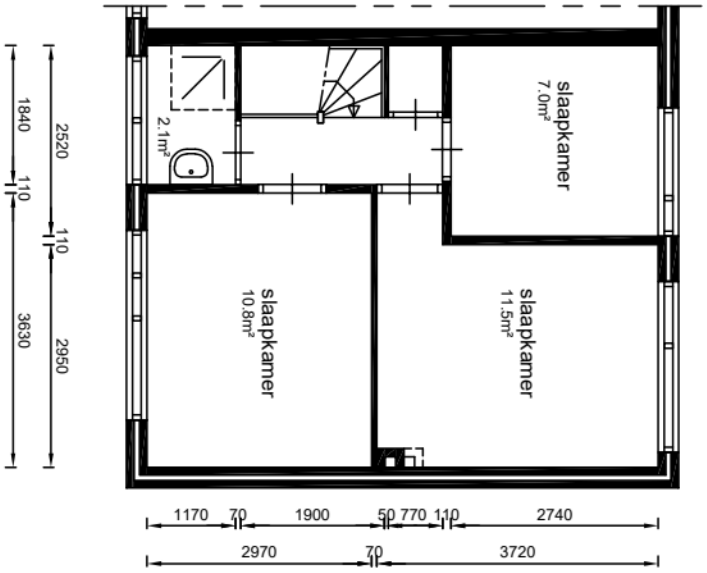
verdieping
