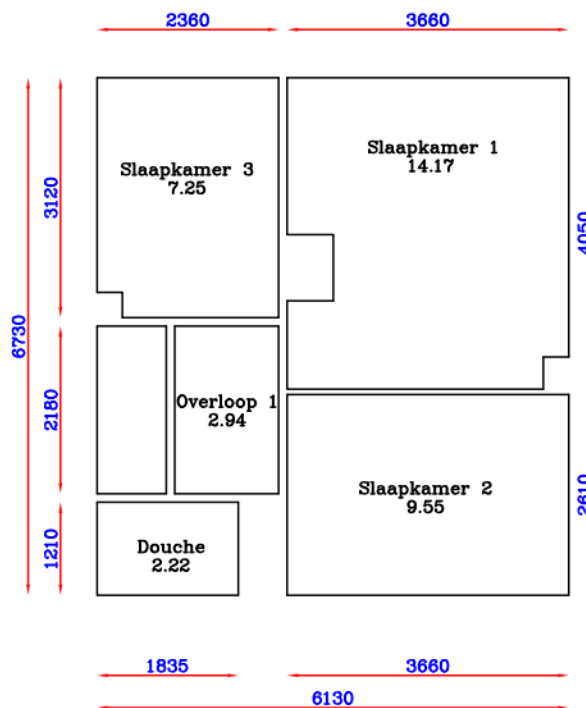
1e Verdieping
