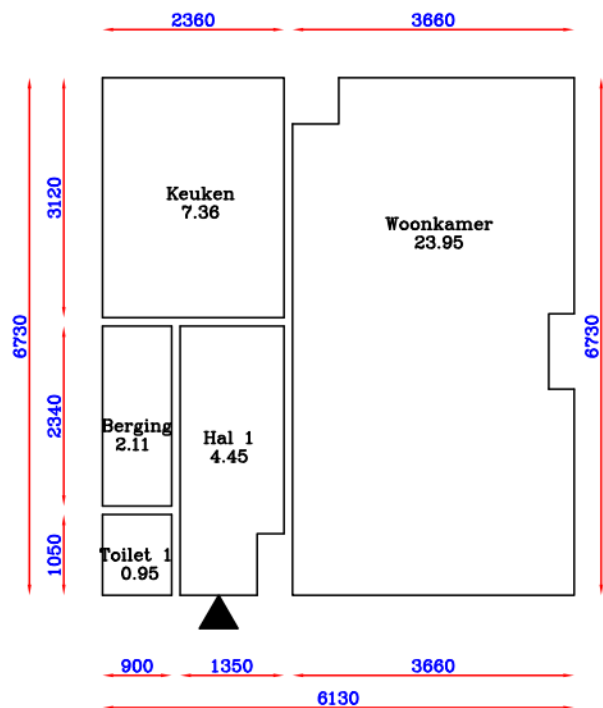
Begane grond
